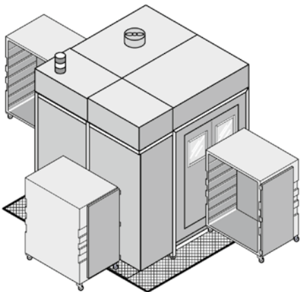
Single-chamber cart washer WWA 15-1K
